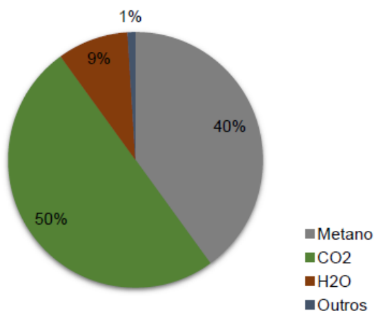
Figura 12: Composição estequiométrica dos gases produzidos no inteiro do maciço de aterros sanitários.
